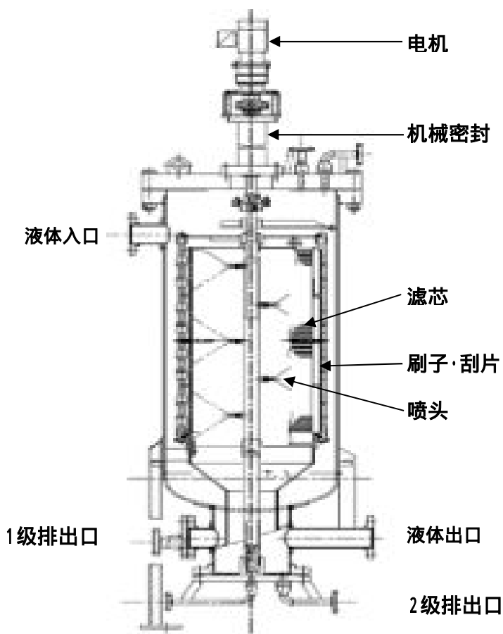
结构图
