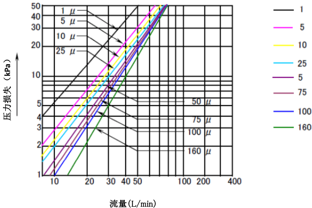
DURACLEAN 通水阻力值 (聚丙烯材, 长250mm滤芯)
